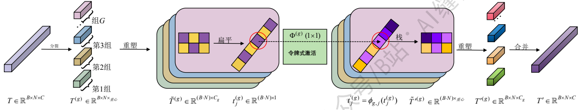
图3: 分组KAN激活示意图。给定标记嵌入 T \in \mathbb{R}^{B \times N \times C} , 我们将通道维度划分为 G 个组, 每个组重塑为 (B \cdot N) \times C_g 。随后对每个组中的每个标量维度独立应用一维KAN函数 \Phi^{(g)} 。输出经过重塑和拼接后, 生成激活表示 T' \in \mathbb{R}^{B \times N \times C} 。
