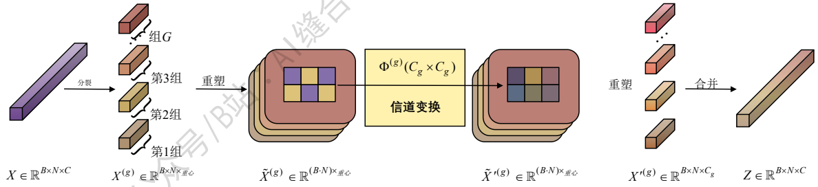
图4: 分组KAN变换示意图。输入特征 X \in \mathbb{R}^{B \times N \times C} 沿通道维度被划分为 G 个组。每个组被重塑为 (B \cdot N) \times C_g , 并通过一个具有可学习映射的非线性变换 \Phi^{(g)} (大小为 C_g \times C_g ) 进行处理。变换后的输出被重塑并拼接, 形成输出 Z \in \mathbb{R}^{B \times N \times C} 。
