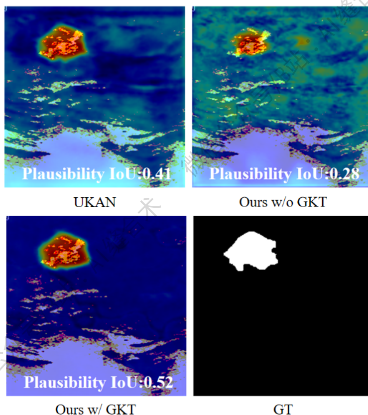
图7: 用于可解释性比较的通道激活图。带 GKT 的GroupKAN（左下）与GT掩码（右下）的对齐效果最佳，达到最高的似然IoU（0.52）。U-KAN和不带 GKT 的GroupKAN对齐效果较差，凸显了 GKT 在提升可解释性方面的作用。
