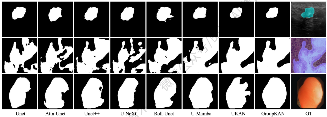
图5: Busi、GlaS与CVC-ClinicDB数据集分割结果的定性对比。GroupKAN在异质性医学影像模态中生成更准确且一致的掩膜，与真实标注高度吻合。
