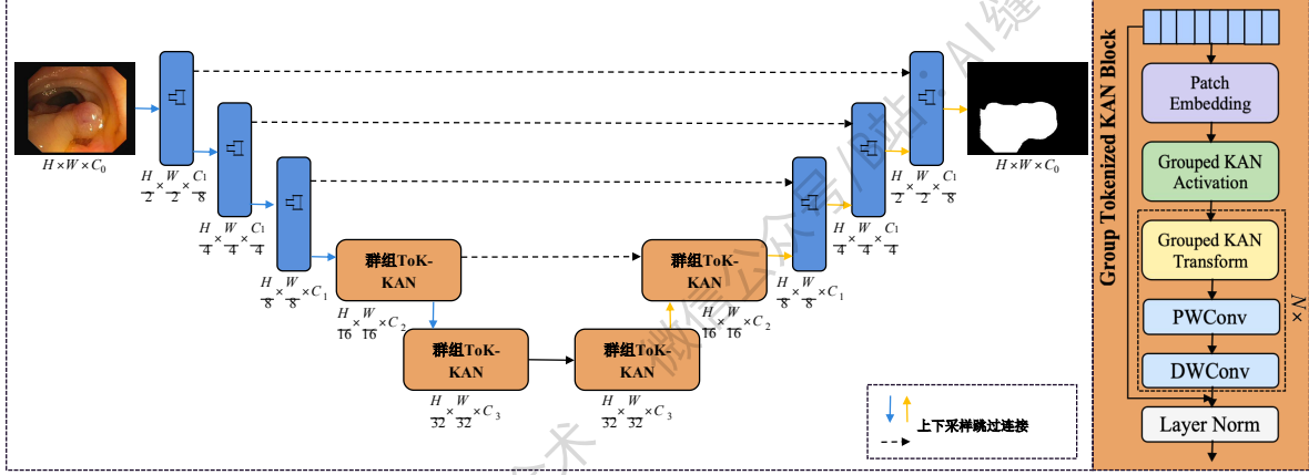
图2: GroupKAN流水线架构示意图。编码器通过卷积模块提取特征。在瓶颈层中, 每个Group ToK-KAN模块依次执行补丁嵌入和分组KAN激活, 随后进行 N 次分组KAN变换, 包含逐点和深度卷积操作。解码器通过上采样和跳跃连接对编码器进行镜像处理, 最终生成分割图。
